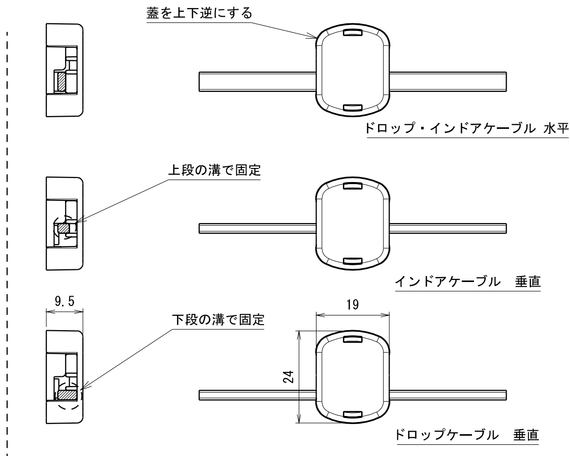
施工パターン図
